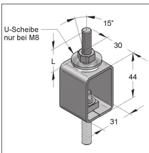
Ingás felfüggesztő
