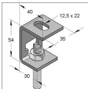
Magasságállítható függesztő T típus
