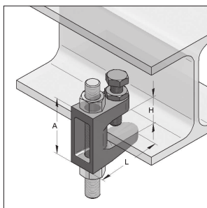
Gerendakapocs TKN öntvény
