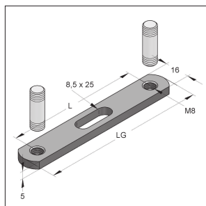
Dupla tartó belső menettel
