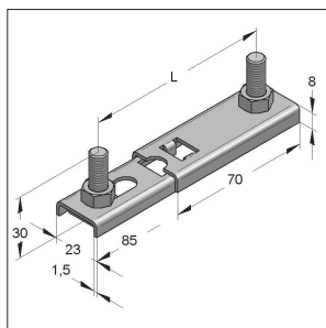
Dupla tartó VS
