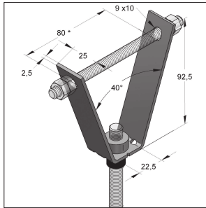
Trapézlemez függesztő magasságbeállítóval
