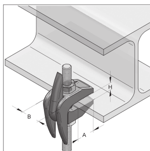
Gerendakapocs F9
