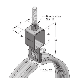
Magasságbeállító
