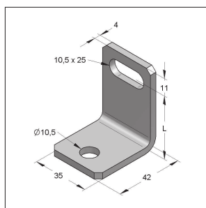
Távtartó sarokelem E
