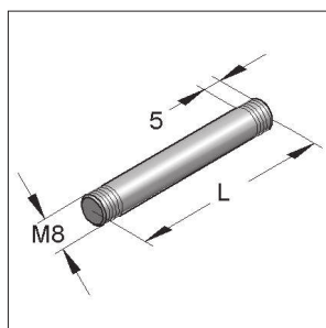
Menetes csap
