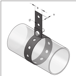
Szerelőszalag - PLA Acél
