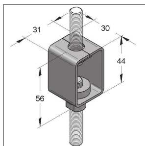
Magasságállító SMU
