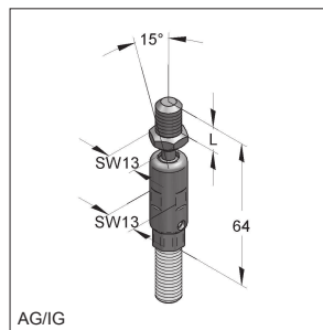
Ingás függesztő M10/M10
