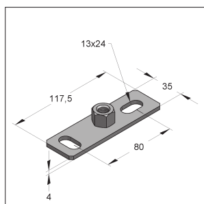
Alaplemez I típus
