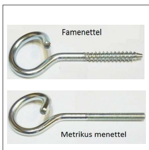
Hintahorog
