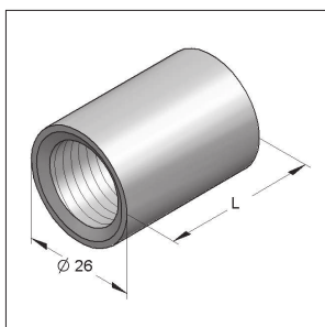
Menetes karmantyú
