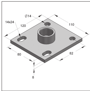
Alaplemez IV típus
