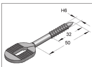
Szemescsavar oválfurattal
