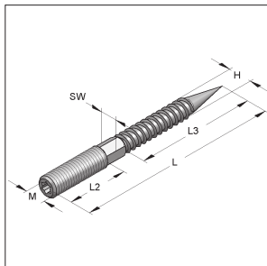
Vállnélküli tőcsavar négyzetes TX 25
