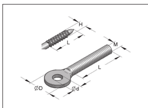
Szemescsavar
