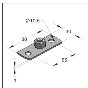
Alaplemez 0 típus
