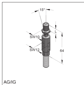
Ingás függesztő M8/M8
