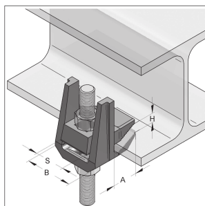
Gerendakapocs F3 kétrészes
