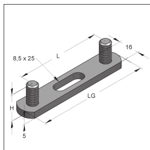
Dupla tartó MD
