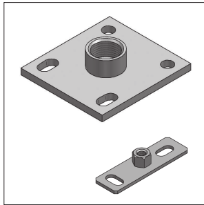
Alaplemez 5/2 oldal
